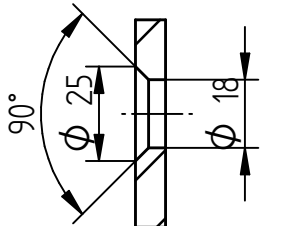
Schnitt A-A
