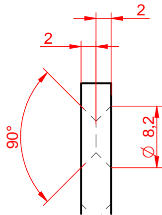
DETALLE A
