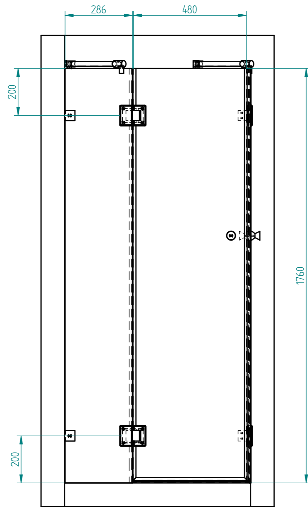
EINZELHEIT H 1:2
