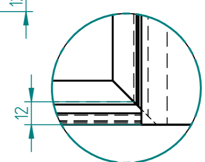
EINZELHEIT F 1:2
