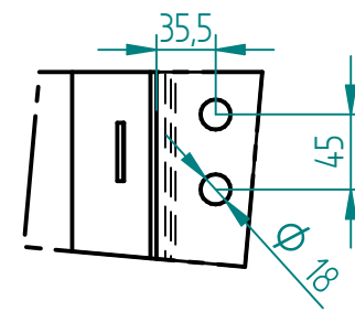
EINZELHEIT E
