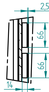
EINZELHEIT C
