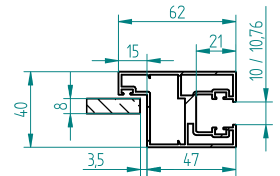
Schnitt A-A
